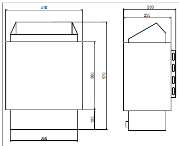
Рис. 5. Размеры электрокаменки
