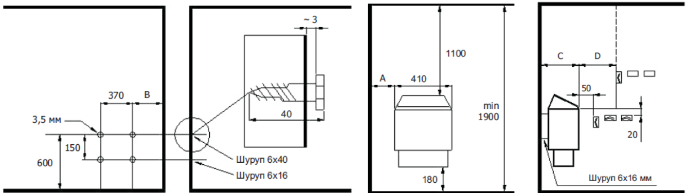
Рис. 1. Схема установки электрокаменки
